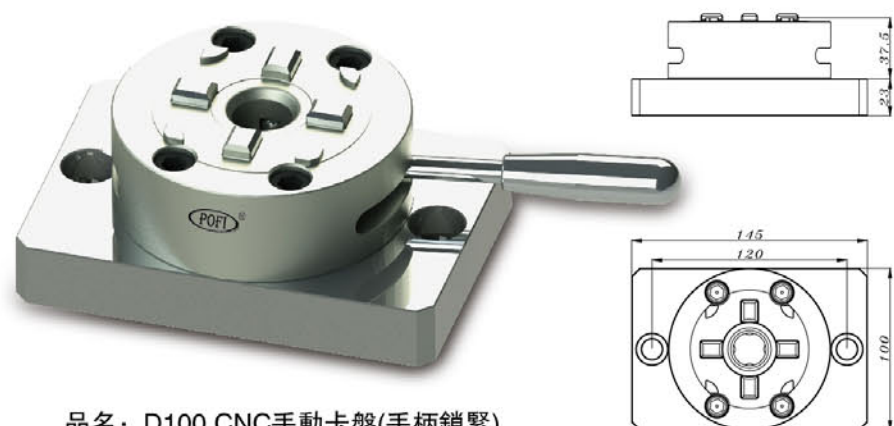
品名: D100 CNC手動卡盤(手柄鎖緊) D100 3M Manual Chuck Wit CNC Base
