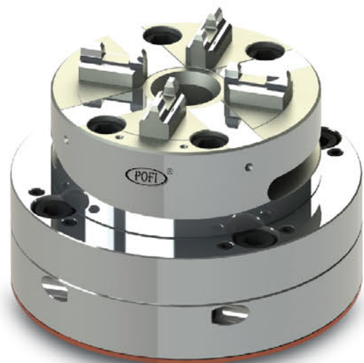
品名: D100 EDM手動卡盤 Manual Chuck D100 With EDM Base
