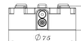
品名：D75手動單頭卡盤（螺絲鎖緊） D75 3M Marco Chuck
