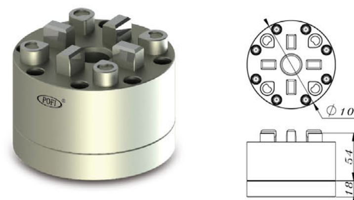
品名: D100 單頭氣動卡盤 D100 3M Pneumatic Chuck
