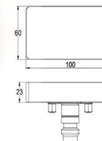
品名：100x60零位基準座 Parallel Gauging Pin
