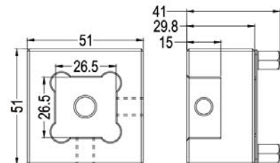
品名: S25方型不銹鋼夾頭 S25 STAINLESS STEEL HOLDER
