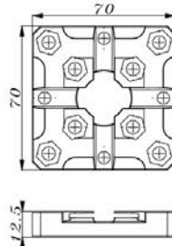
品名: 70x70定位片 3M Centering Plate 70x70
