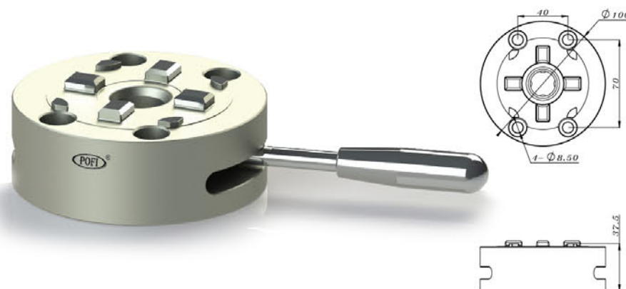
品名: D100單頭手動卡盤(手柄鎖緊) D100 3M Manual Chuck
