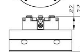
品名：D75 EDM手動卡盤（螺絲鎖緊） D75 3M EDM Marco Chuck
