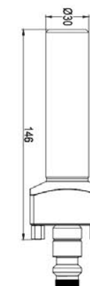
品名： \Phi 30 柱型零位基準座 Checking Pin
