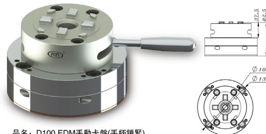
品名: D100 EDM手動卡盤(手柄鎖緊) D100 3M Manual Chuck Wit EDM Base
