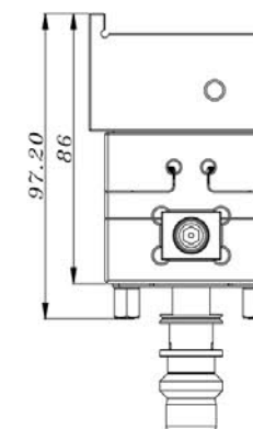
品名：3向微調線切割夾具 3 Axes High Precision Control Jig
