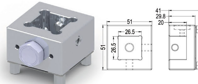
品名: S25槽型鋁合金夾頭 S25 ALUMINUM HOLDER
