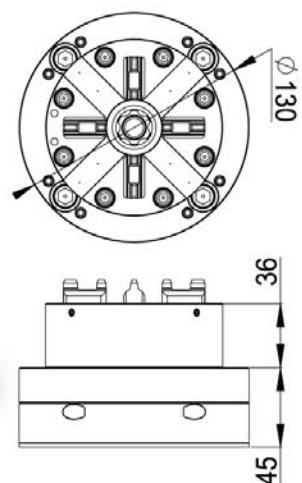
品名: D100 EDM氣動卡盤 EDM PNEUMATIC CHUCK D100
