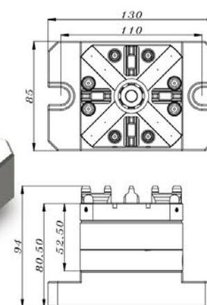
品名: 80方型CNC氣動卡盤 80 mm Square CNC Pneumatic Chuck
