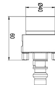
品名：50x50零位基準座 Gauging Pin
