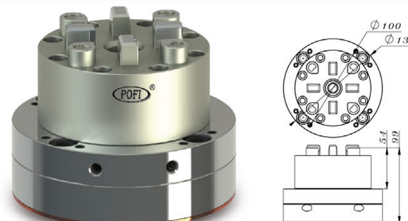
品名: D100 EDM氣動卡盤 D100 3M EDM Pneumatic Chuck
