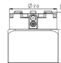
品名：D75 CNC手動卡盤（螺絲鎖緊） D75 3M CNC Marco Chuck
