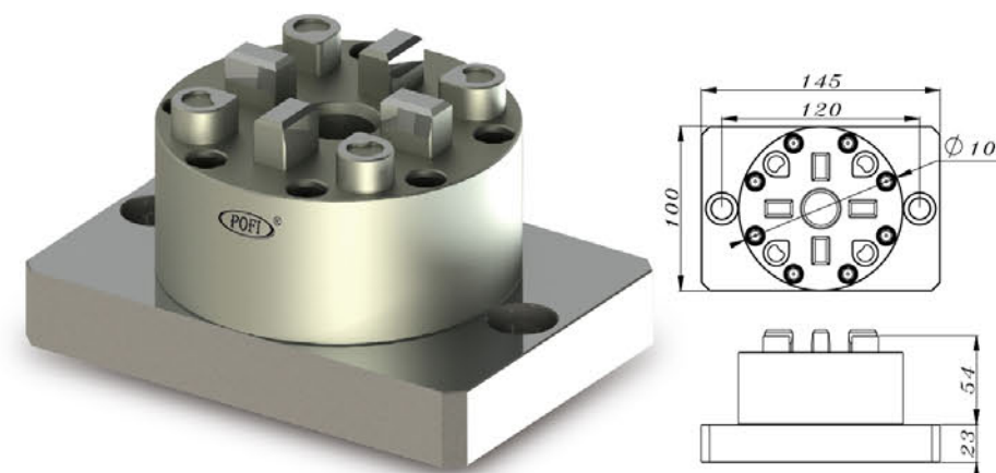
品名: D100 CNC氣動卡盤 D100 3M CNC Pneumatic Chuck
