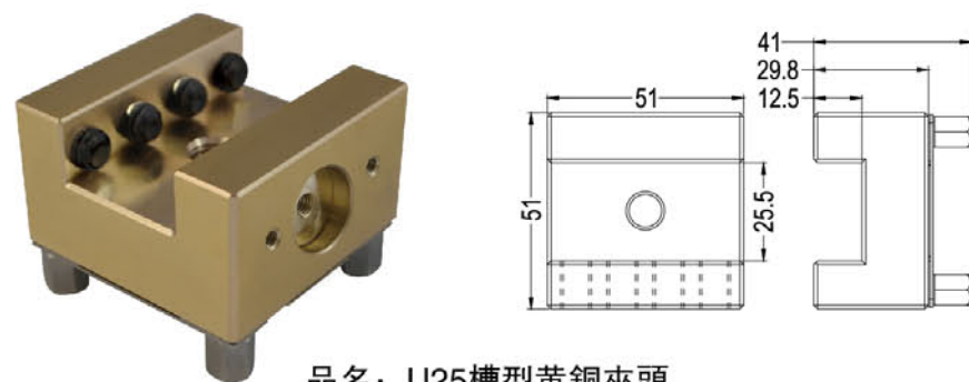
品名: U25槽型黃銅夾頭 U25 BRASS HOLDER
